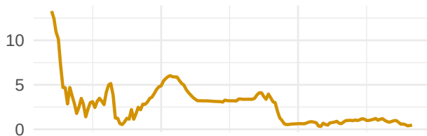
m2_gap
