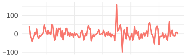
igae
