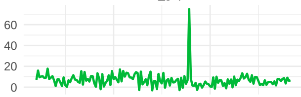
pi_crb
